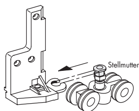
Bild 1 Stellmutter in richtige Position bringen und Laufwagen einschieben
